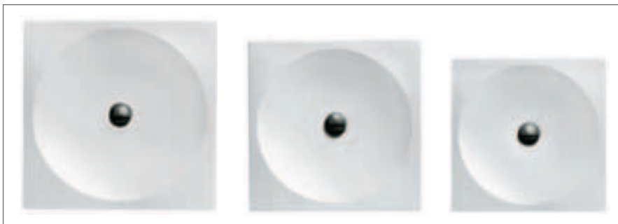
Quadrat-Brausewanne Ohne Styropor-Wannenträger 1.000 x 1.000 x 45 mm Modell K 6704 xx*
