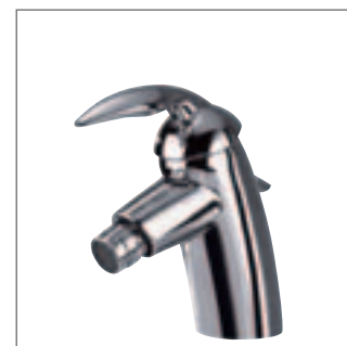
Bidetarmatur Ausladung 108 mm Auslaufhöhe 58 mm Modell A 3003 xx*
