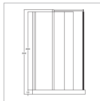
Duschabtrennung 90 1.400 x 895 x 2.060 mm Sicherheitsglas 6 mm, Konstruktion und Profile Aluminium verchromt, für linke und rechte Raumecke, passend zur Brausewanne L 5238 01 und L 5237 01 L 8376 AA
