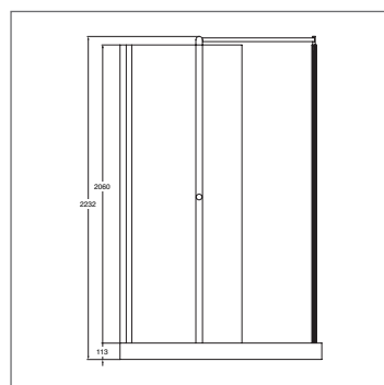
Duschabtrennung 180 1.400 x 845 x 2.060 mm Sicherheitsglas 6 mm, Konstruktion und Profile Aluminium verchromt, für linke und rechte Raumecke, passend zur Brausewanne L 5236 01 und L 5235 01 L 8374 AA
