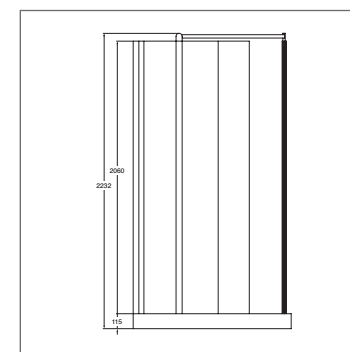
Duschabtrennung 90 1.200 x 895 x 2.060 mm Sicherheitsglas 6 mm, Konstruktion und Profile Aluminium verchromt, für linke und rechte Raumecke, passend zur Brausewanne L 5240 01 und L 5239 01 L 8378 AA
