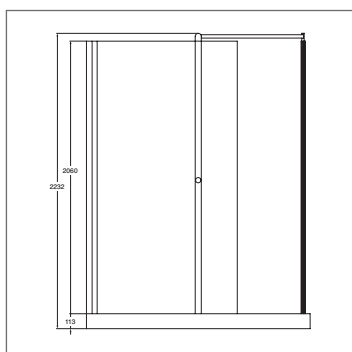
Duschabtrennung 180 1.700 x 845 x 2.060 mm Sicherheitsglas 6 mm, Konstruktion und Profile Aluminium verchromt, für linke und rechte Raumecke, passend zur Brausewanne L 5234 01 und L 5233 01 L 8368 AA
