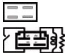
12V/20A
