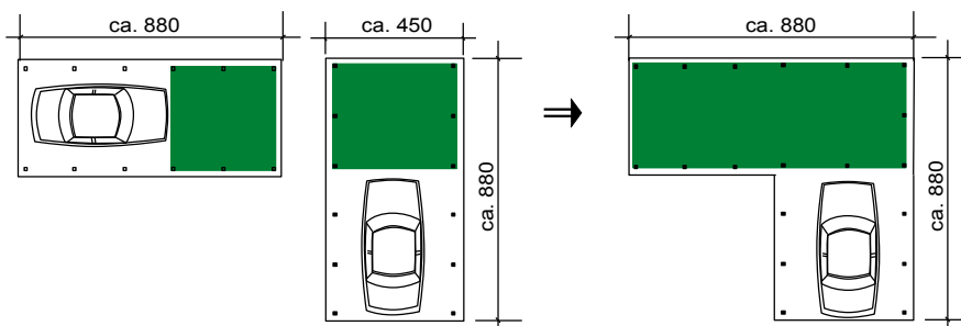
Aus Zwei mach Eins. Zwei lange Carports über Eck kombiniert.
