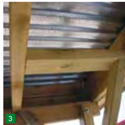
3 Kopfband-Wechsel – er dient zwischen den Pfetten als Anschlagpunkt für das Quer-Kopfband.
