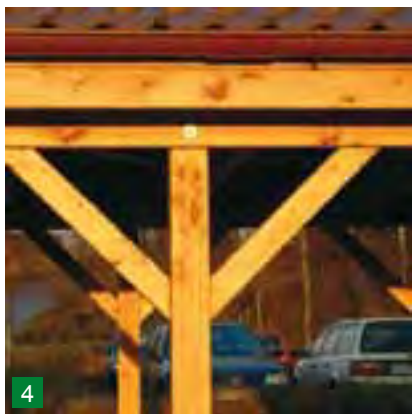
4 Längs-Kopfband links und rechts. Statisch bedeutend als Aussteifung Ihres Carports in Längsrichtung.
