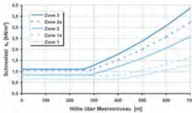
Charakteristischer Wert der Schneelast für Geländehöhe und Schneelastzone nach DIN 1055-5
