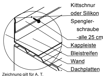
Carport als Wandanbau-Variante – „Bergen MWT“, Natur-Serie, hier: wandseitig mit Pfosten.
