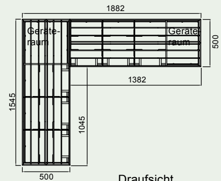
Draufsicht
