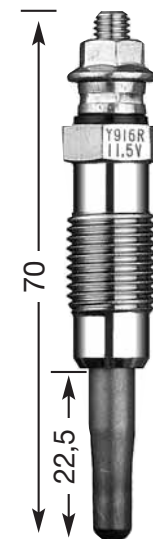
Y-916 R M 12 x 1.25 12 Hex 11,5 V DP 6
