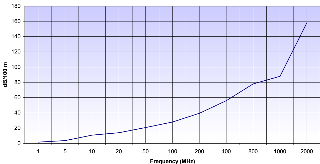
Attenuation
