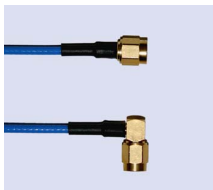
Kabel / Cable Anschluß Connector Multiflex 86 SMA-Stecker/SMA-Winkelstecker SMA male/SMA angle male
