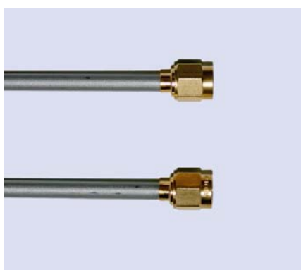
Kabel / Cable Anschluß Connector Semi Rigid UT 141 TP SMA-Stecker/SMA-Stecker SMA male/SMA male
