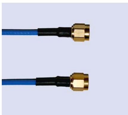
Kabel / Cable Anschluß Connector Multiflex 141 SMA-Stecker/SMA-Stecker SMA male/SMA male
