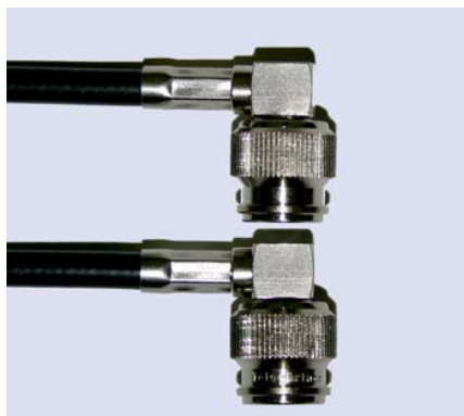
Kabel / Cable Anschluß Connector RG58C/U TNC-Winkelstecker/TNC-Winkelstecker TNC angle male/TNC angle male
