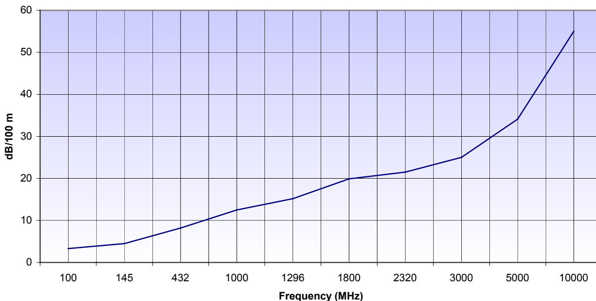
Attenuation
