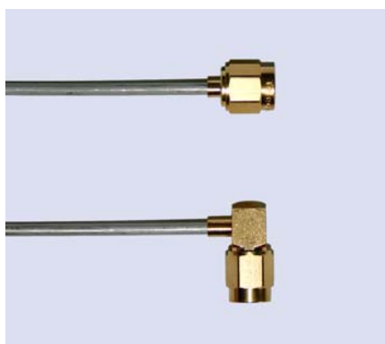
Kabel / Cable Anschluß Connector Semi Rigid UT 85 TP SMA-Stecker/SMA-Winkelstecker SMA male/SMA angle male
