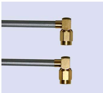
Kabel / Cable Anschluß Connector Semi Rigid UT 141 TP SMA-Winkelstecker/SMA-Winkelstecker SMA angle male/SMA angle male
