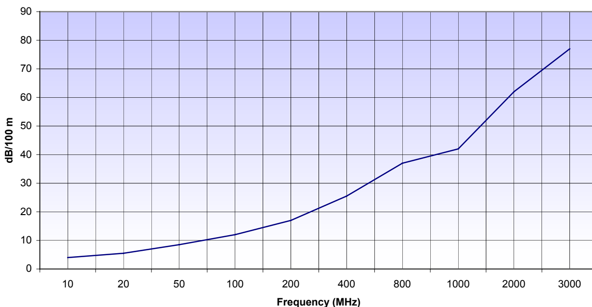
Attenuation
