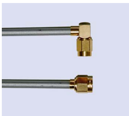
Kabel / Cable Anschluß Connector Semi Rigid UT 141 TP SMA-Winkelstecker/SMA-Stecker SMA angle male/SMA male
