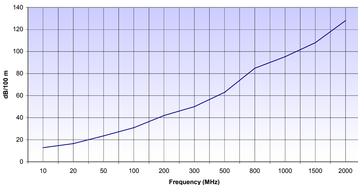
Attenuation
