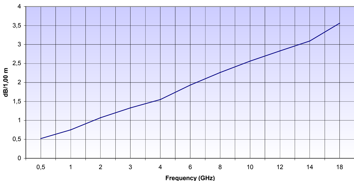
Attenuation
