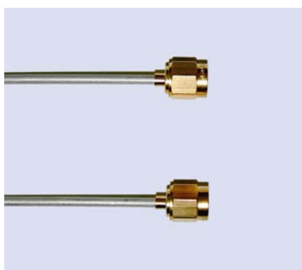
Kabel / Cable Anschluß Connector Semi Rigid UT 85 TP SMA-Stecker/SMA-Stecker SMA male/SMA male
