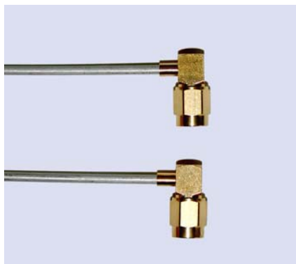
Kabel / Cable Anschluß Connector Semi Rigid UT 85 TP SMA-Winkelstecker/SMA-Winkelstecker SMA angle male/SMA angle male
