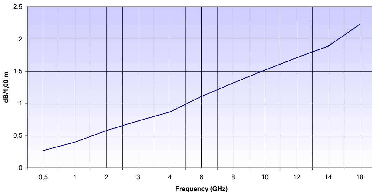
Attenuation
