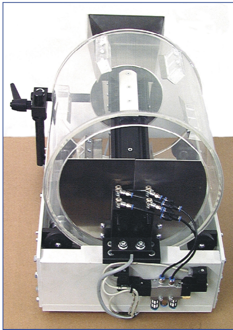
Mehrbahniges Federentwirr- und Zuführsystem Trommelförderer TF 300 B
