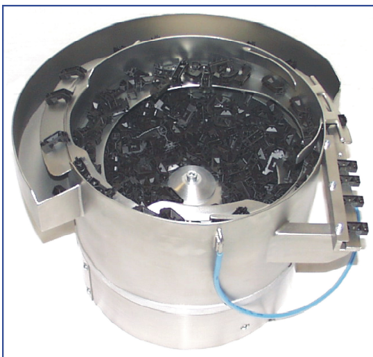
Kohlenbürstengehäuse Leistung: 30 Teile pro Minute Teilesortierung: Ausführung V2A
