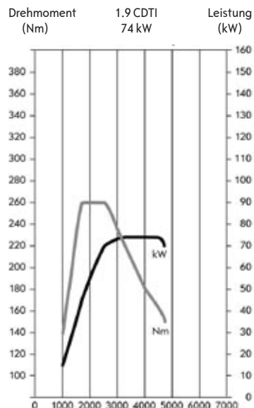
Motordrehzahl (min -1 )
