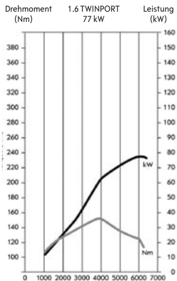
Motordrehzahl (min -1 )
